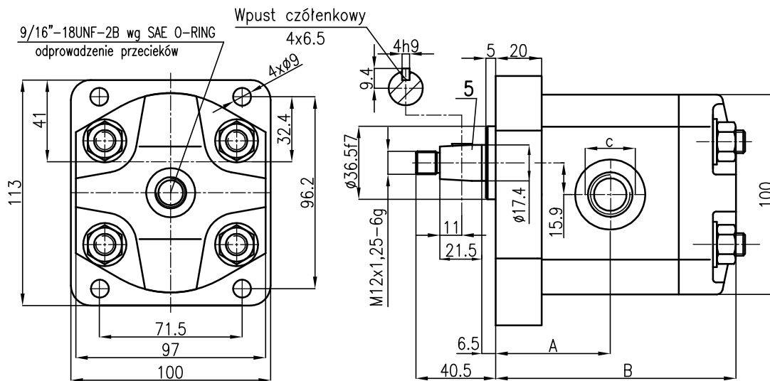
5 -czop stożkowy 1:8
